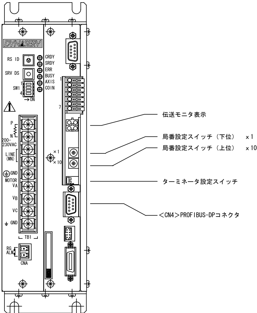
PROFIBUS-DPインタフェース フロントパネル
