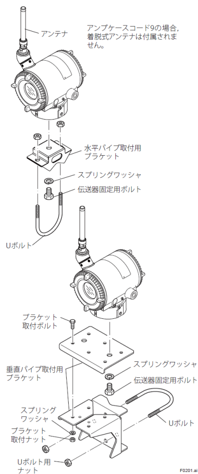
図 2.1 伝送器取付用部品
