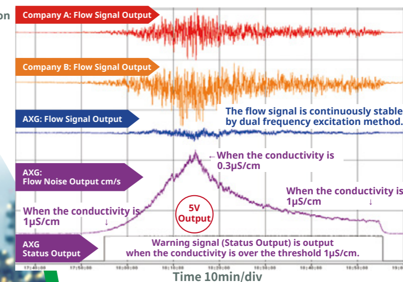
Time 10min/div
