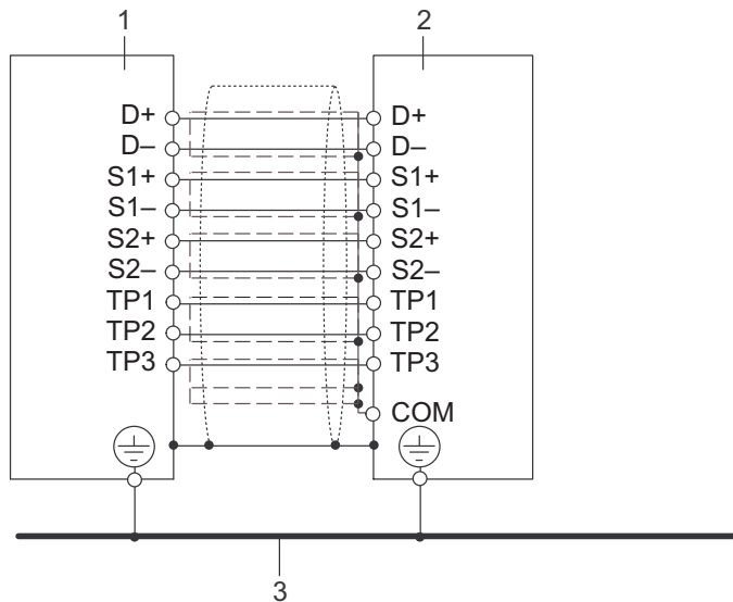
Рис. 26. Схема электрических соединений измерительного преобразователя и датчика
