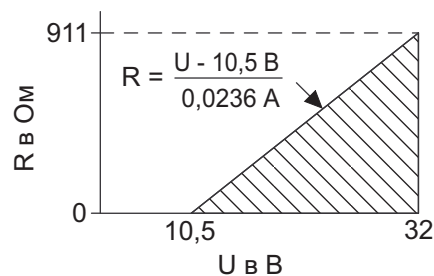
Рис. 32. Зависимость максимального сопротивления нагрузки от напряжения внешнего источника питания
