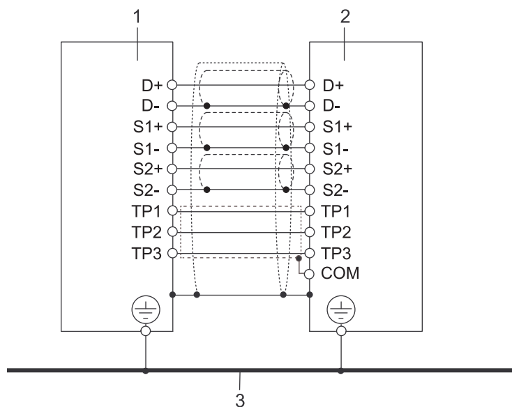
Рис. 24. Схема электрических соединений измерительного преобразователя и датчика
