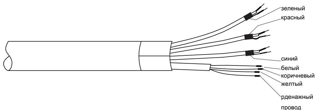
Рис. 25. Стандартный соединительный кабель с концевой заделкой L 100 , сторона измерительного преобразователя
