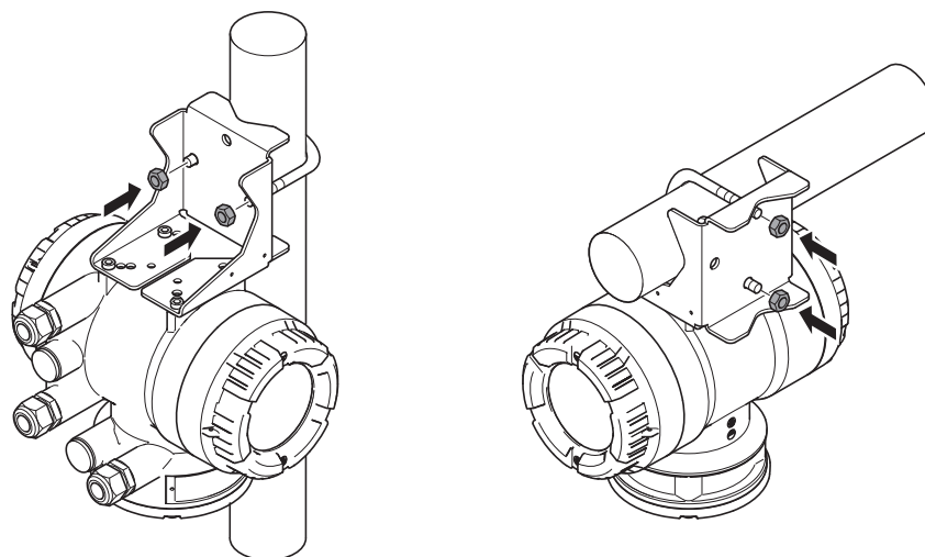
Рис. 9. Подвешивание дистанционного измерительного преобразователя
