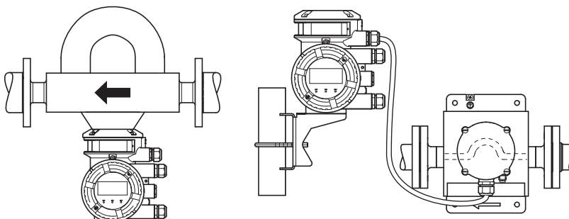
Рис. 5. Горизонтальный монтаж, измерительные трубки вверх
