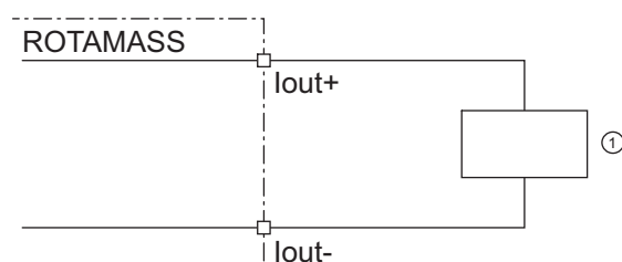
Рис. 31. Соединение активного токового выхода I out HART
