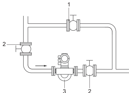
Рис. 2. Запорные клапаны и байпасная линия
