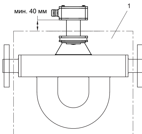
Рис. 19. Изоляция, поставляемая заказчиком
