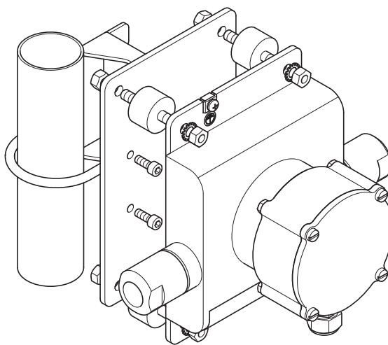
Рис. 17. 2-дюймовое крепление, опция /PD для Nano
