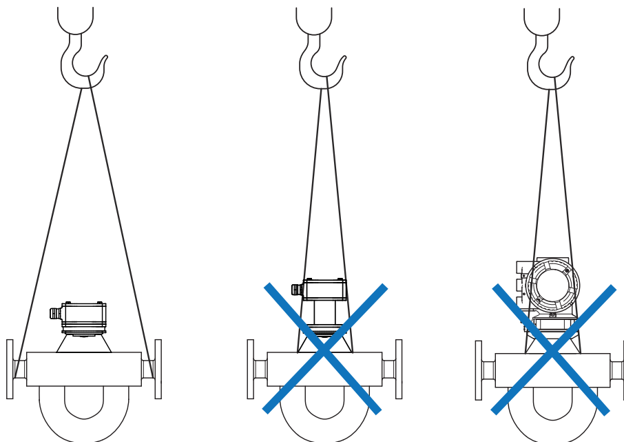
Рис. 1. Крепление транспортировочных тросов к датчику независимо от конструкции (недопустимые способы крепления зачеркнуты)
