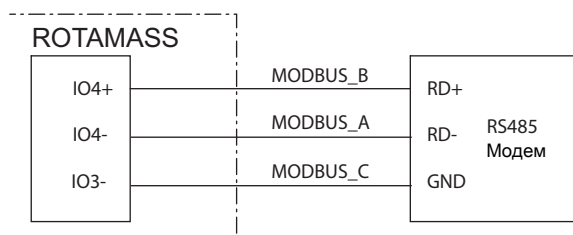
Рис. 29. Связь по протоколу MODBUS
