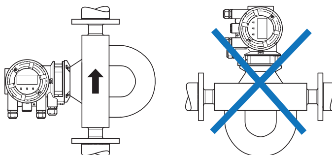
Рис. 8. Положение при установке, соответствующее нормам EHEDG
