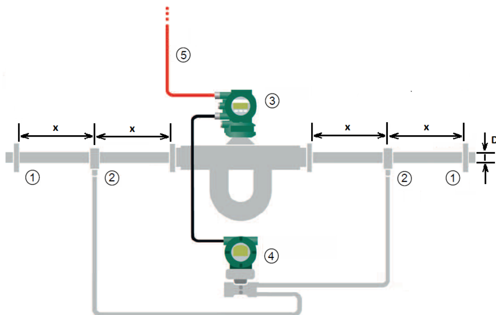
Рис. 18. Размещение точек измерения давления
