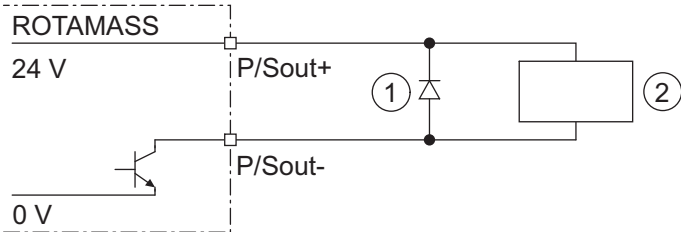
Рис. 35. Соединение активного импульсного выхода P/Sout с электромеханическим счетчиком
