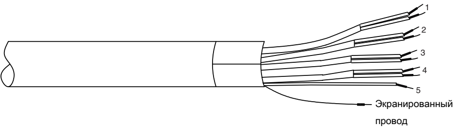
Рис. 27. Огнестойкий соединительный кабель с концевой заделкой Y UL , сторона измерительного преобразователя
