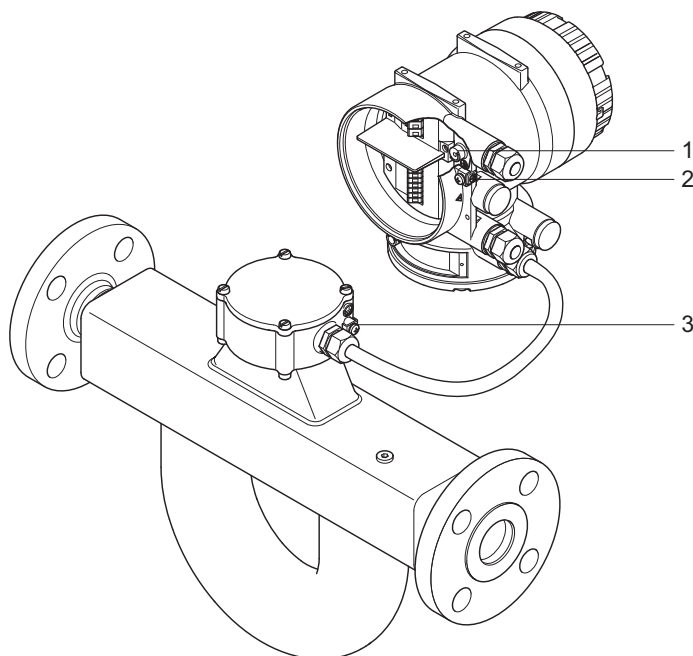
Рис. 20. Подключение заземления на измерительном преобразователе и датчике
