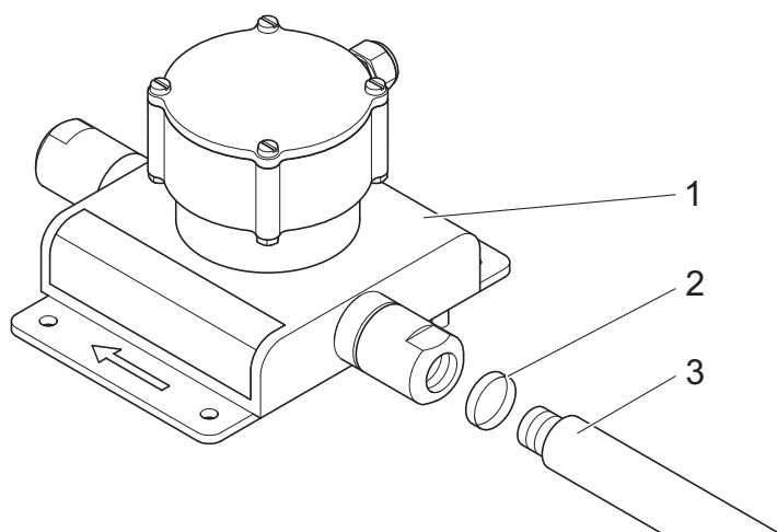
Рис. 16. Внутреннее резьбовое соединение
