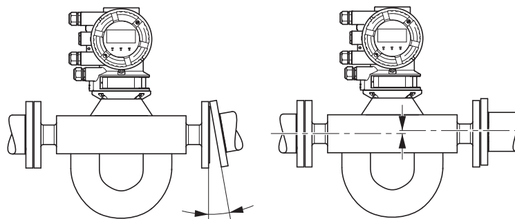
Рис. 12. Избегайте: уклона и перекося
