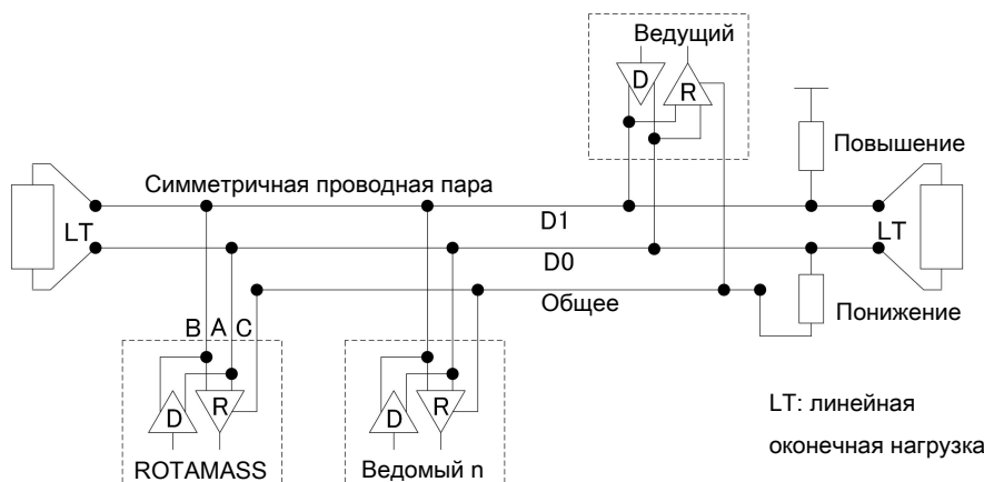
Рис. 30. Соединение Modbus
