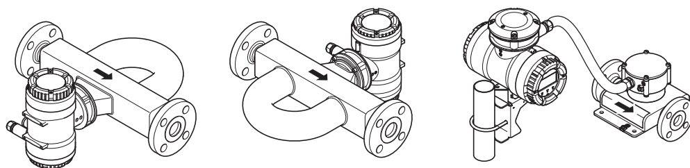
Рис. 3. Нежелательные положения при установке: Расходомер в наклонном положении
