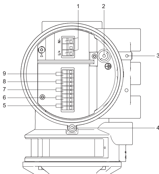
Рис. 28. Клеммная коробка для выходов I/O и источника питания измерительного преобразователя
