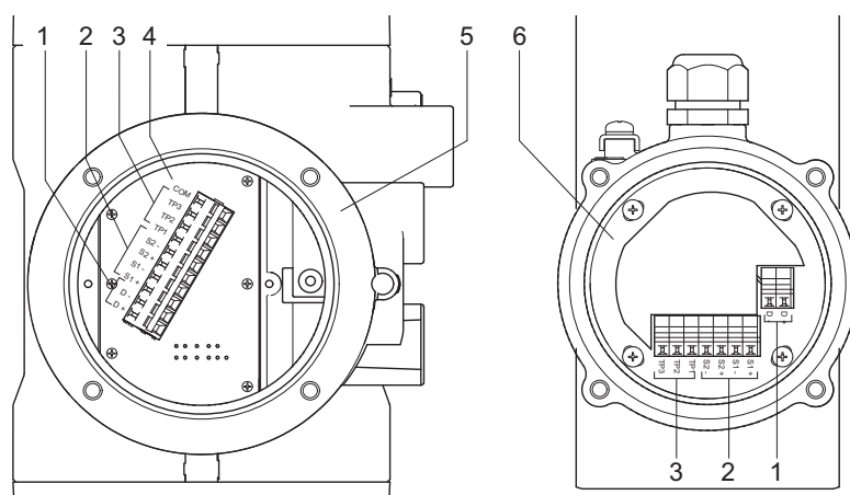
Рис. 21. Цепи соединительных клемм (измерительный преобразователь с левой стороны, датчик с правой стороны)
