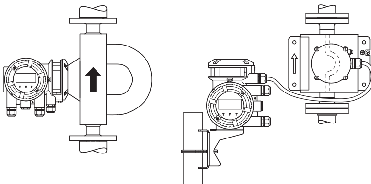
Рис. 7. Вертикальный монтаж
