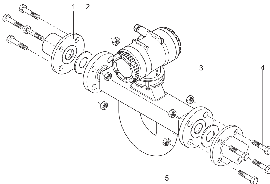
Рис. 15. Крепление фланца
