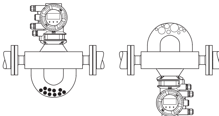
Рис. 6. Опасность скопления твердых частиц и/или газа
