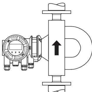
Рис. 10. Вертикальная установка (самодренирование)
