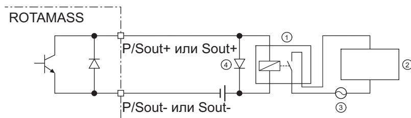
Рис. 42. Соединение пассивного выхода состояния P/Sout или Sout для цепи электромагнитного клапана
