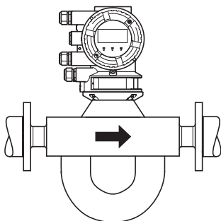
Рис. 11. Горизонтальная установка с трубками внизу
