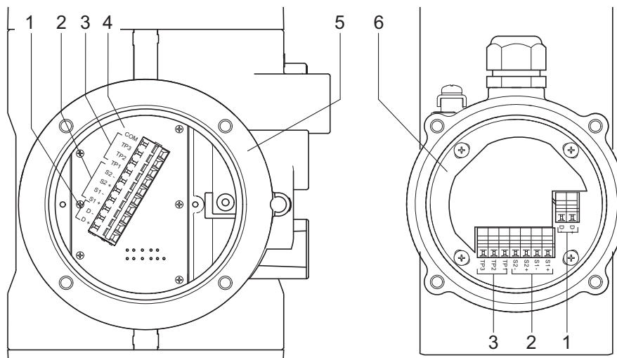
Рис. 23. Цепи соединительных клемм (измерительный преобразователь с левой стороны, датчик с правой стороны)
