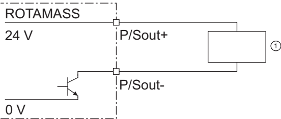
Рис. 39. Соединение активного выхода состояния P/Sout
