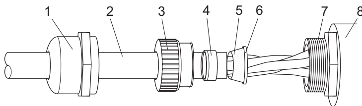
Рис. 22. Монтаж деталей кабельного ввода
