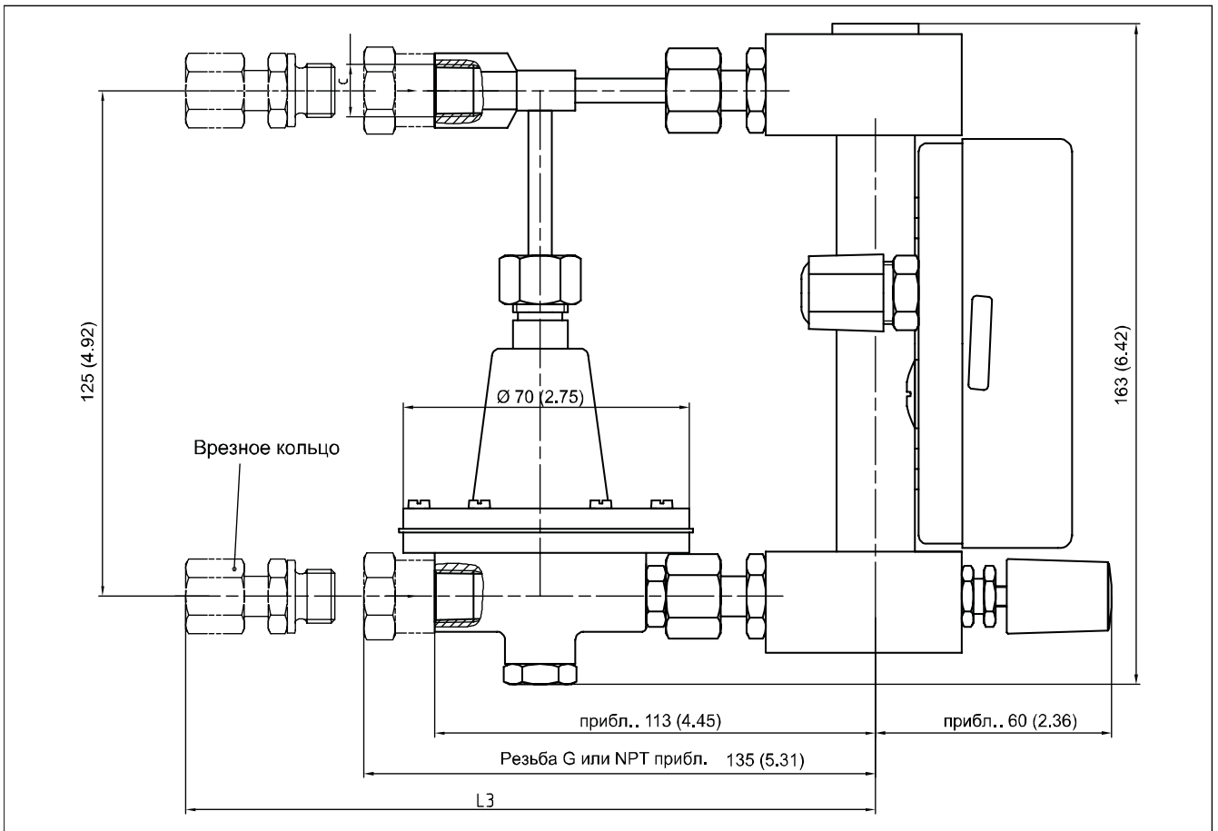
Рисунок 8. Исполнение с впускным клапаном и регулятором впуска
