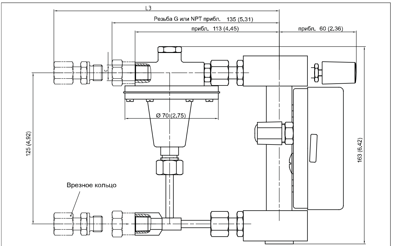
Рисунок 9. Исполнение с выпускным клапаном и регулятором противодействия
