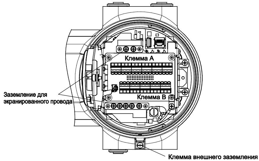
Увеличенная клемма А
