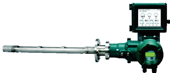
TDLS8200 с блоком ЧМИ YH8000
