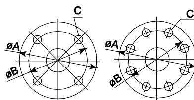
Фланец
