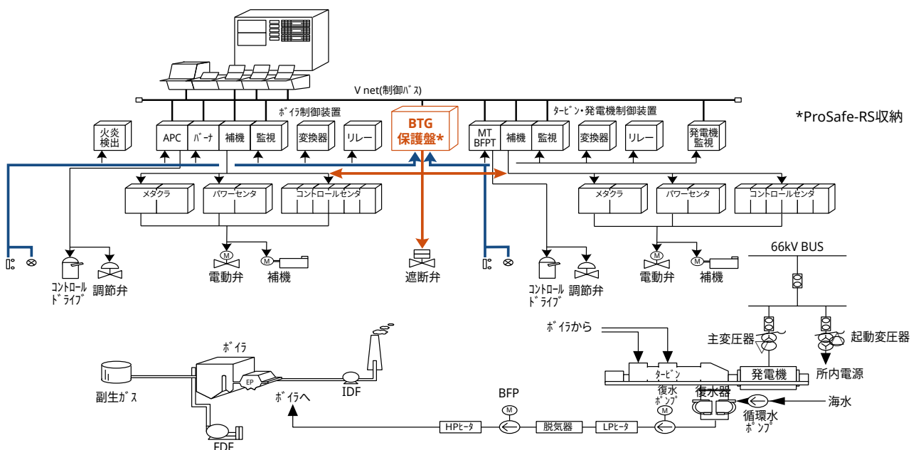
ボイラ・タービン・発電機制御装置システム構成図
