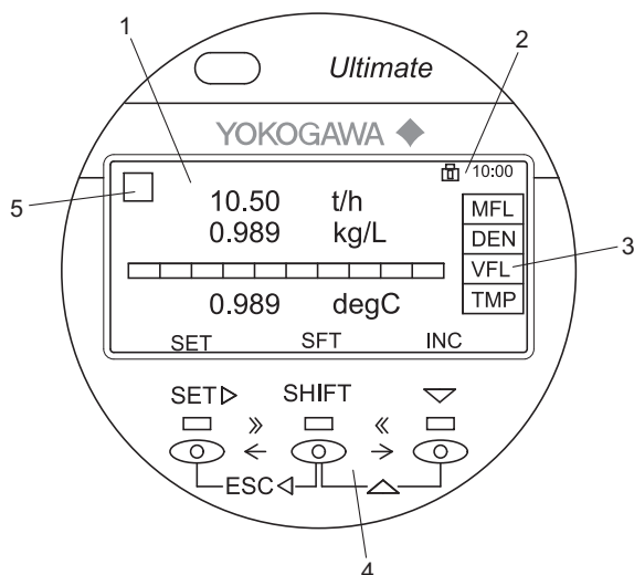
Fig. 46: Display layout
