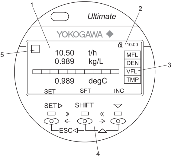
Fig. 37: Display layout
