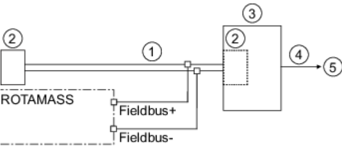
Fig. 37: PROFIBUS PA connection
