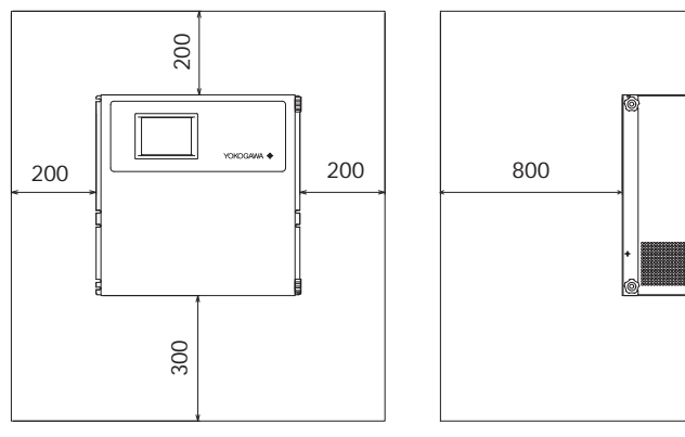
メンテナンススペース
