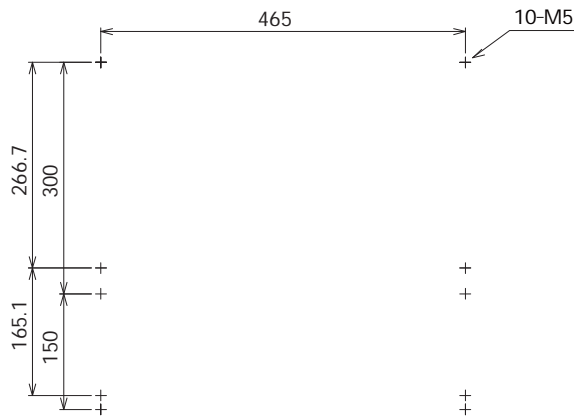
取り付け穴ピッチ
